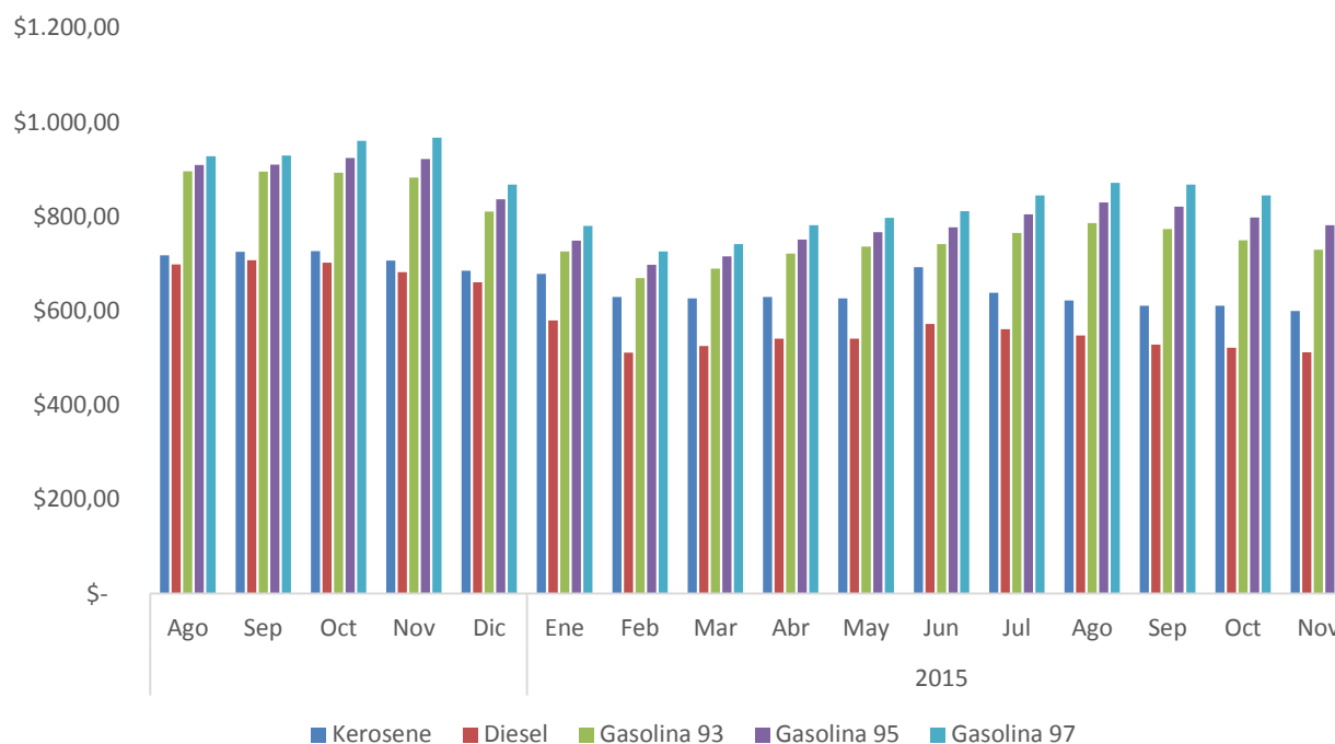
Fig. 3: Evolución del Precio de los distintos tipos de combustibles en la Región de La Araucanía. Agosto 2014 a Noviembre 2015
