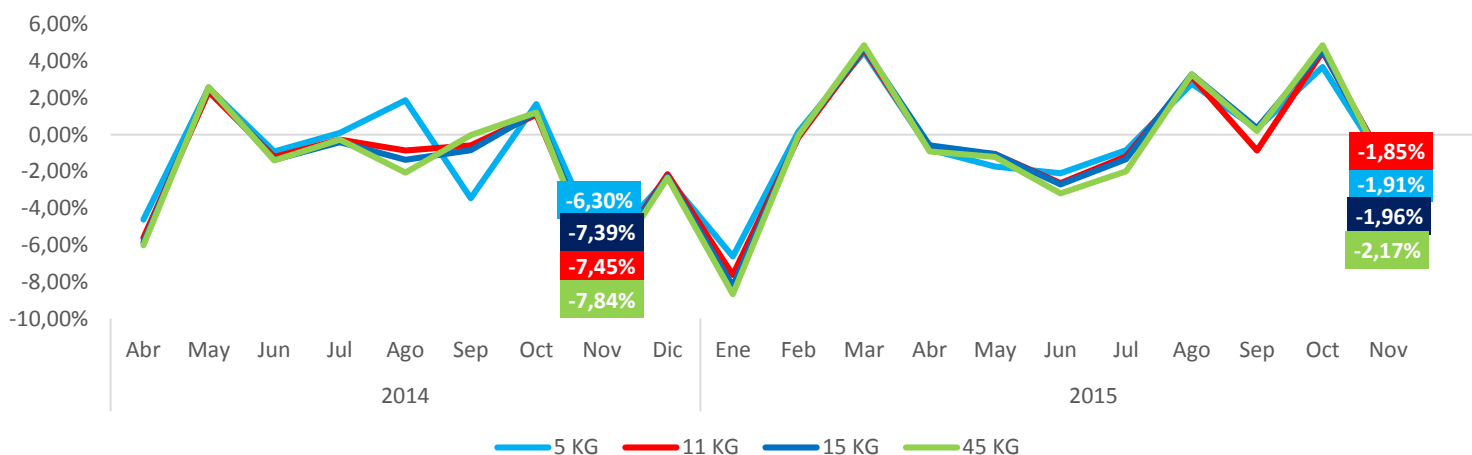
Fig. 5: Variación Mensual del Precio de los distintos tipos de Gas Licuado en la Región de La Araucanía. Abril 2014 a Noviembre 2015
