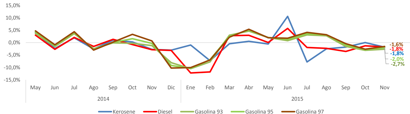
Fig. 2: Variación Mensual del Precio de los distintos tipos de combustibles en la Región de La Araucanía. Mayo 2014 a Noviembre 2015
