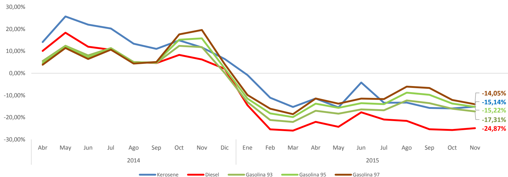
Fig. 1: Variación Anual del Precio de los distintos tipos de combustibles en la Región de La Araucanía. Abril 2014 a Noviembre 2015
