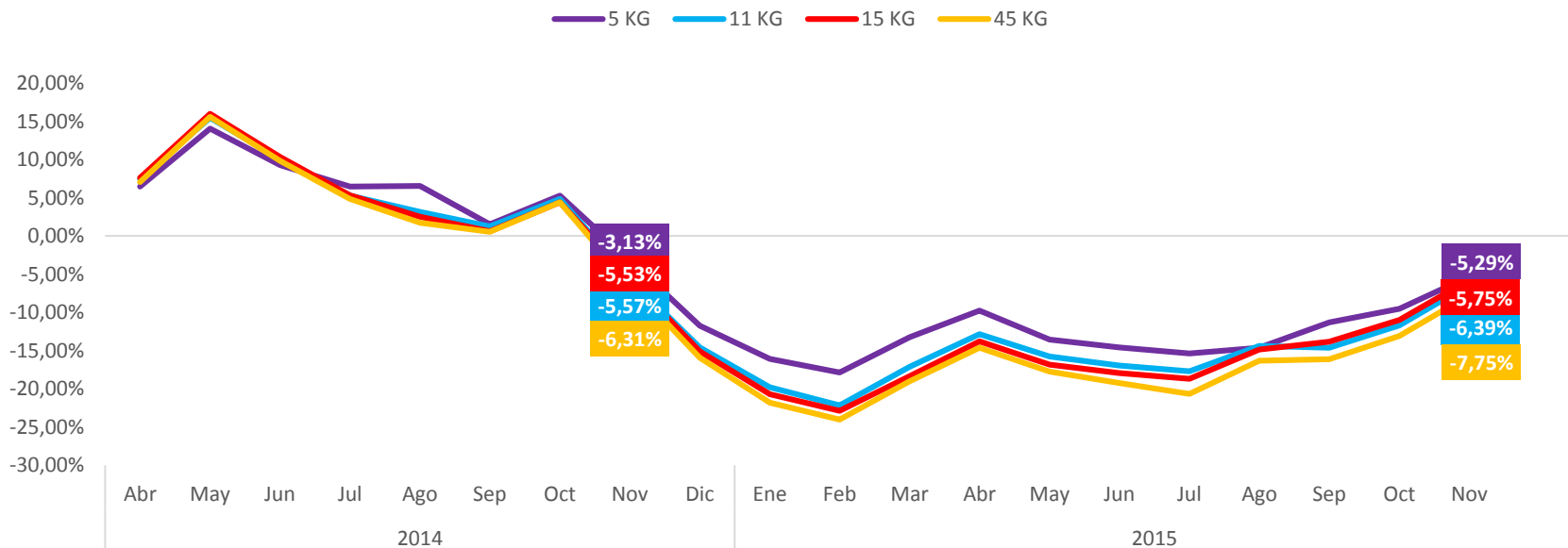
Fig. 4: Variación Anual del Precio de los distintos tipos de Gas Licuado en la Región de La Araucanía. Abril 2014 a Noviembre 2015
